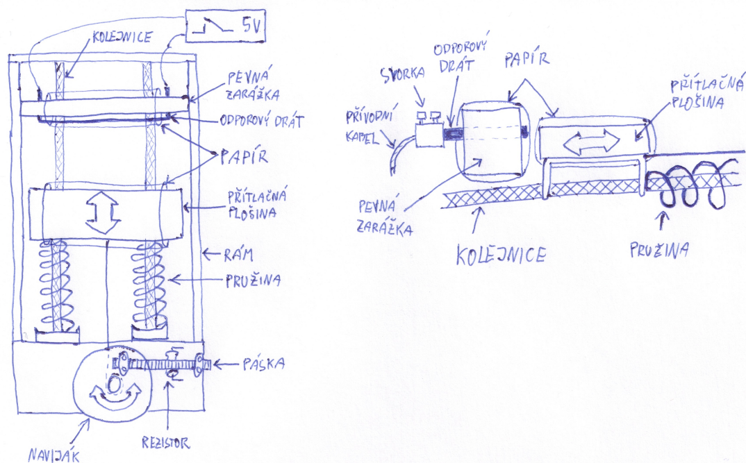
Obrázek 6: Nákres uzavíracího mechanismu balónu
