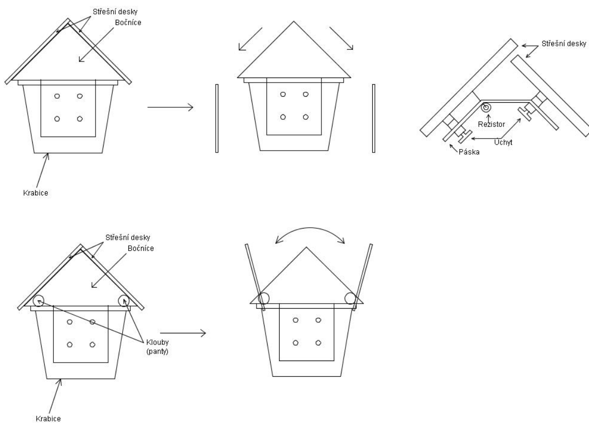
Obrázek 5: Otevírání střechy
