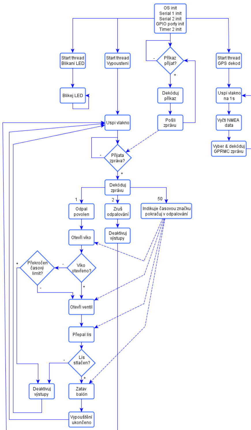
Obrázek 13: Funkční diagram firmwaru Automatického vypouštěče
