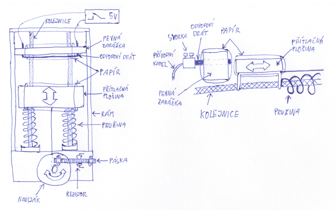
Obrázek 6: Náčrt uzavíracího mechanismu balónu
