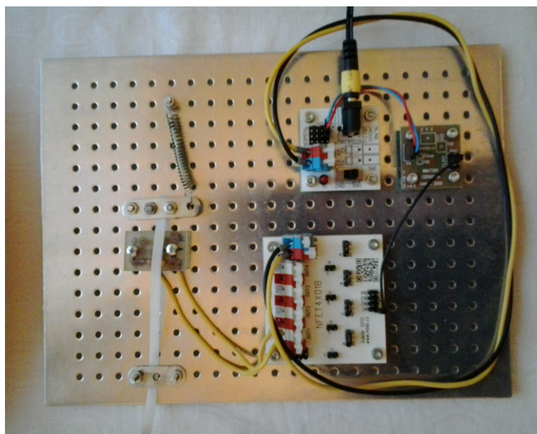
Obrázek 1: Odpalovač víka
