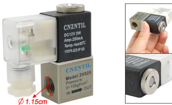
Obrázek 8: Elektromagnetický dávkovací ventil
