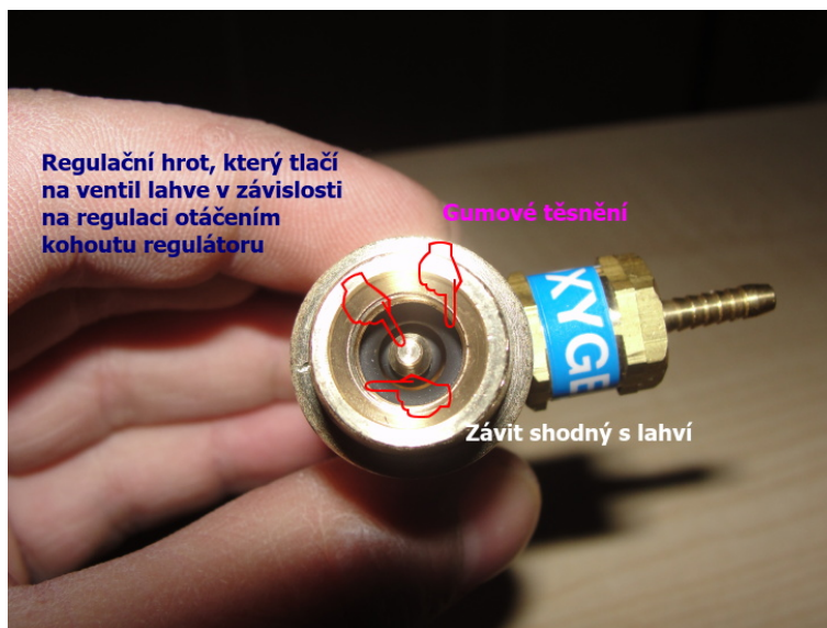
Obrázek 6: Redukční ventil
