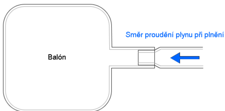
Obrázek 10: Zpětný ventil v nohavici balónu
