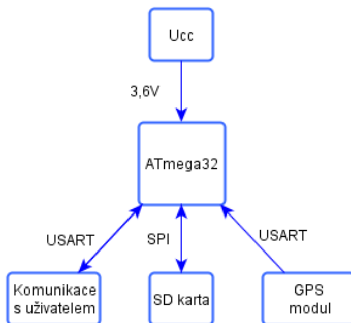
Obrázek 6: Blokové schéma balónové sondy
