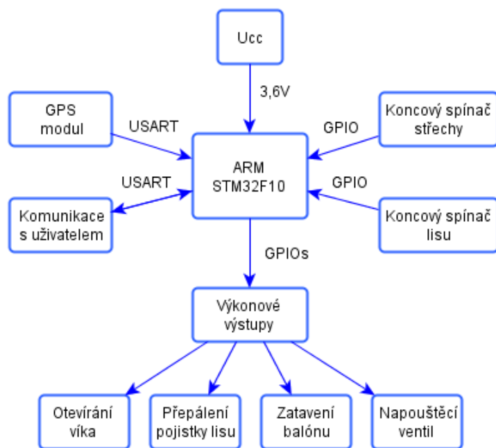
Obrázek 5: Blokové schéma pozemního vypouštěcího boxu
