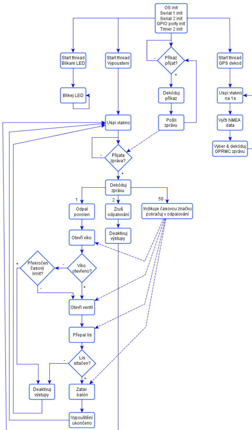
Obrázek 4: Funkční diagram firmwaru Automatického vypouštěče
