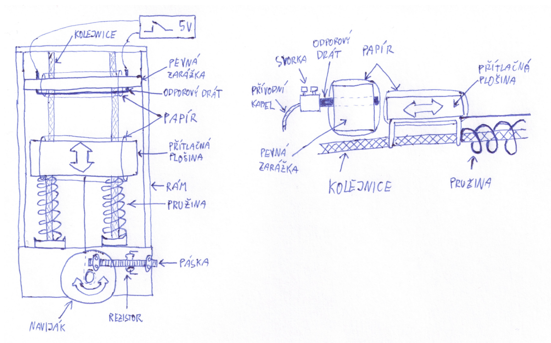
Obrázek 3: Nákres uzavíracího mechanismu balónu
