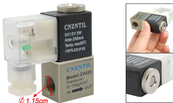
Obrázek 9: Elektromagnetický dávkovací ventil
