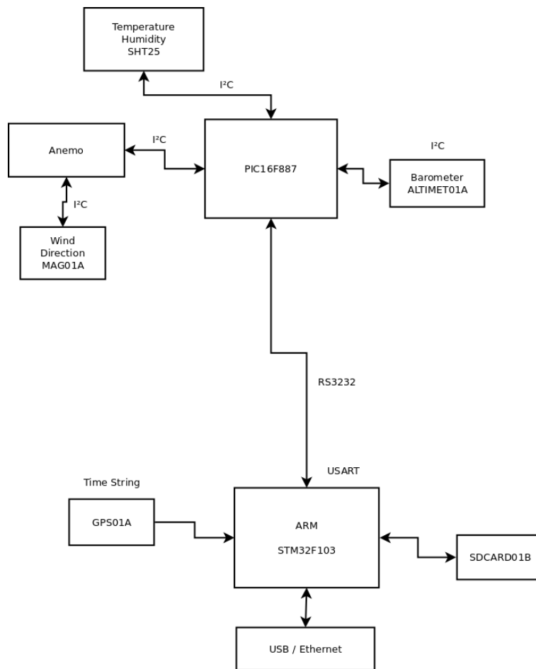
Obrázek 5: Blokové schéma celé konstrukce meteostanice
