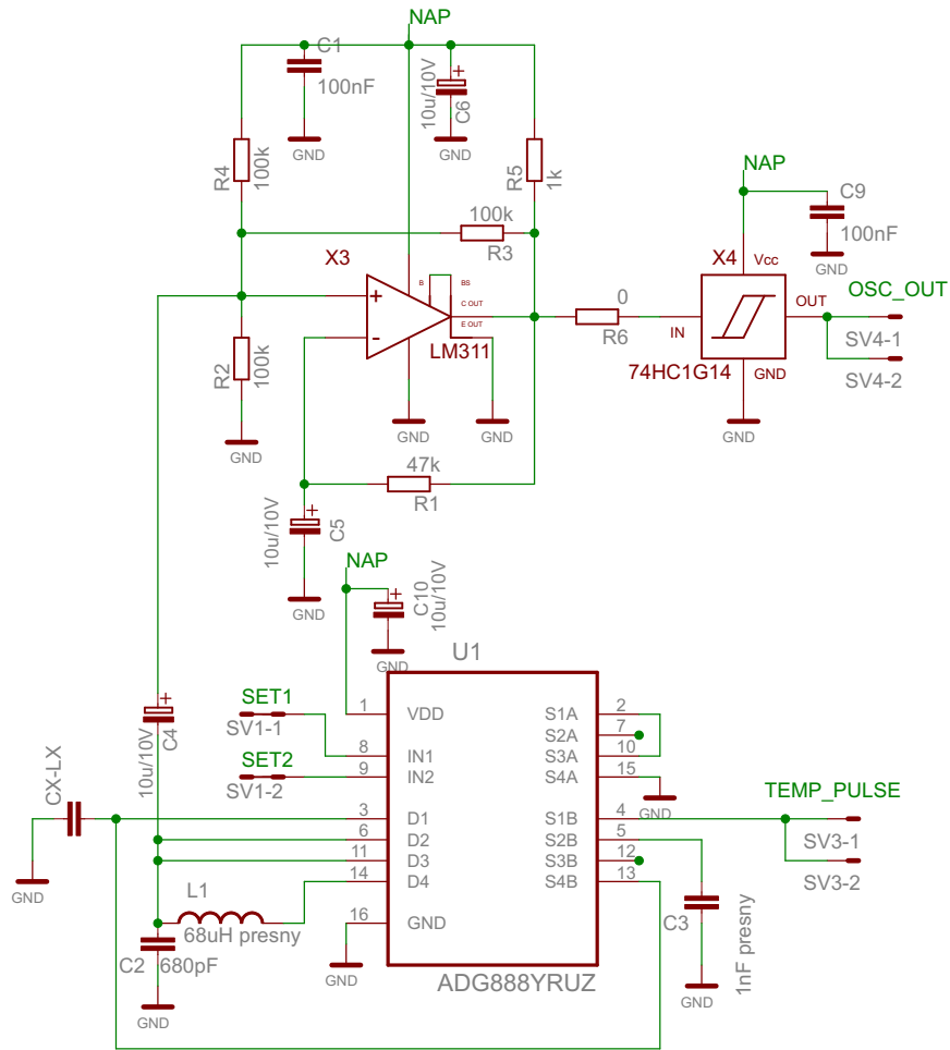
L1 - ELJFA680JFD
