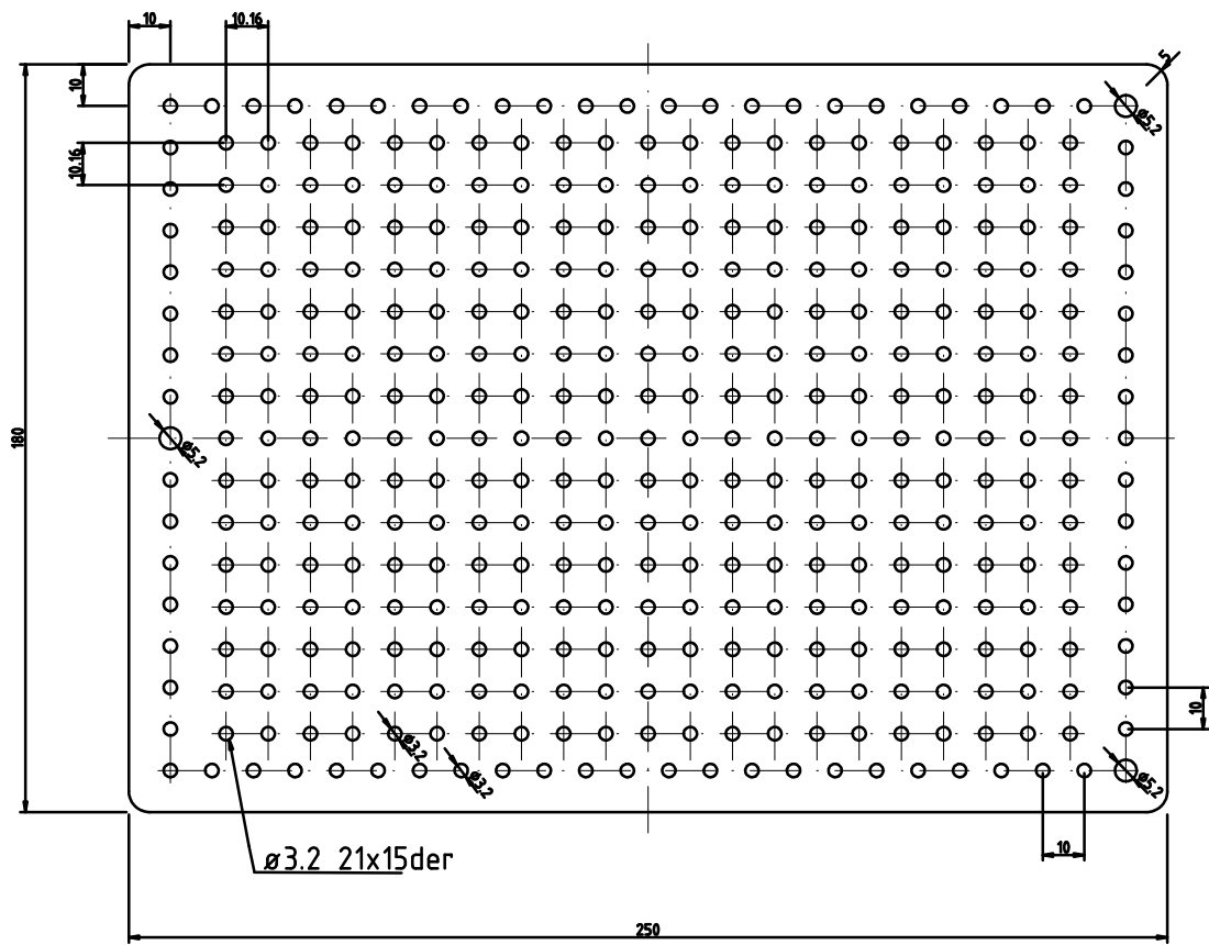
Meritko 1:2
