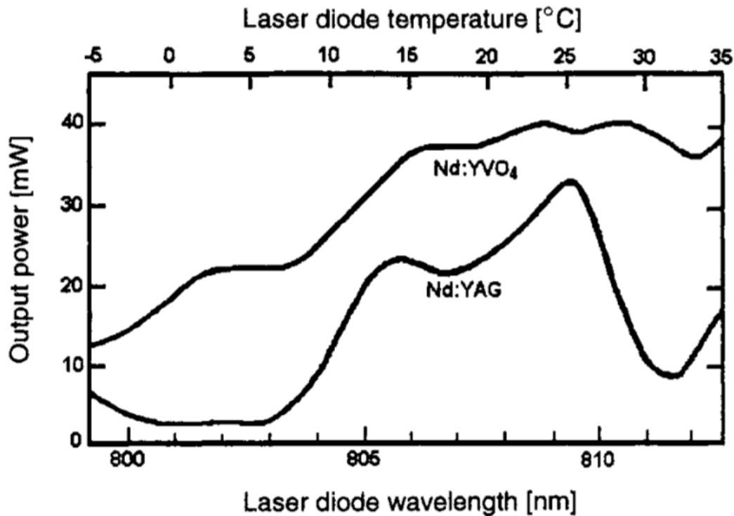
Obrázek 3.2: Výstupní výkon typického \text{Nd:YVO}_4 laseru v závislosti na teplotě diody a vlnové délce [4].
