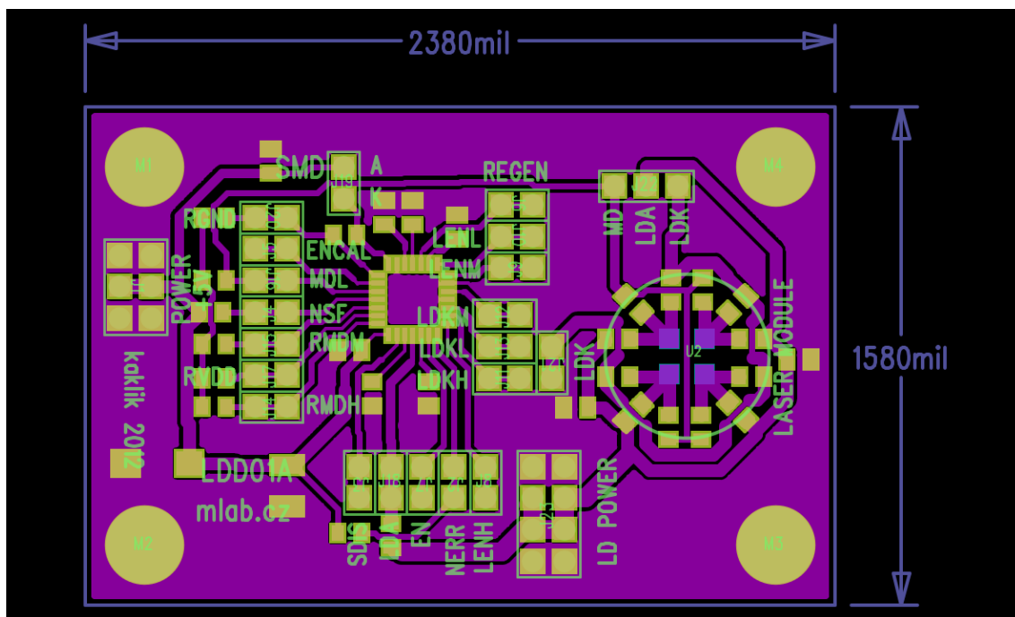
Obrázek 3.13: Návrh plošného spoje pulsního budiče LDD01A
