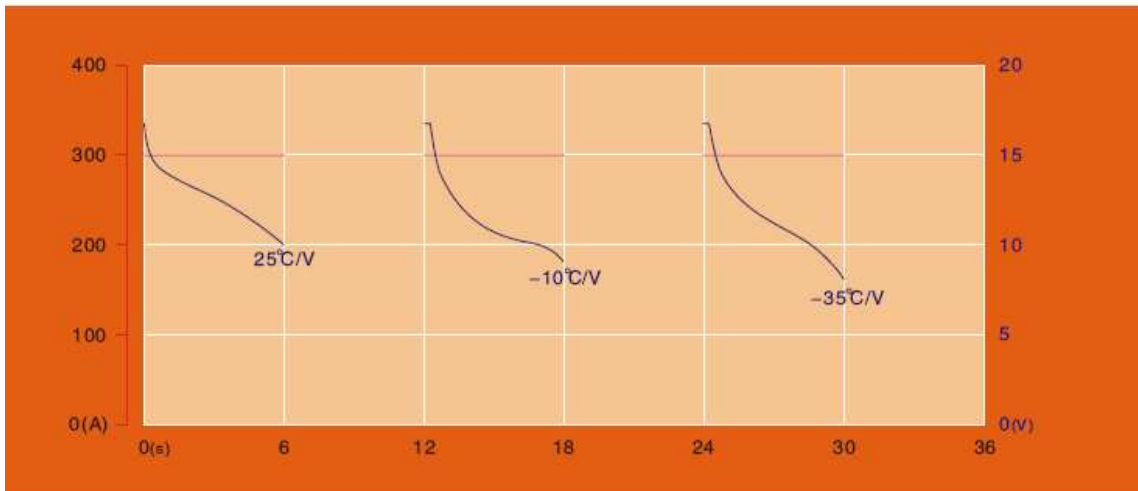
▲ TS-LP12V40AH在不同溫度環境下的脈衝放電特性 TS-LP12V40AH IMPULSE DISCHARGE AT DIFFERENT TEMPERATURE
