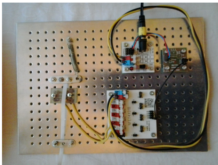
Obrázek 2: Testovací prototyp zajišťovacího mechanismu
