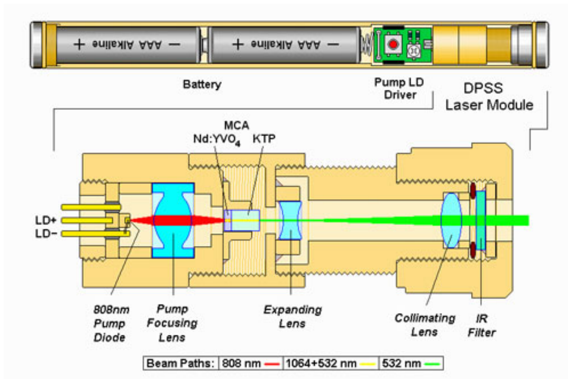
Obrázek 3.2: Typická konstrukce diodově čerpaného pevnolátkového laseru používaného, jako zelené laserové ukazovátko. [1]
