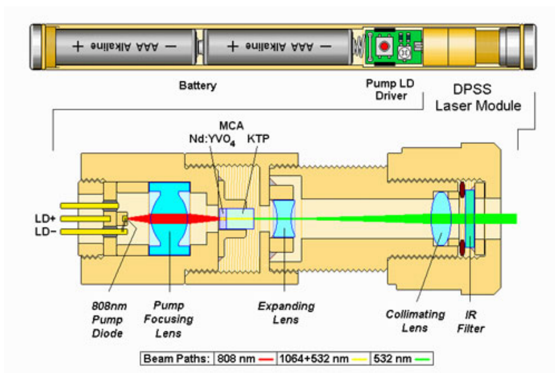
Obrázek 3.1: Typická konstrukce diodově čerpaného pevnolátkového laseru používaného, jako zelené laserové ukazovátko. [?]
