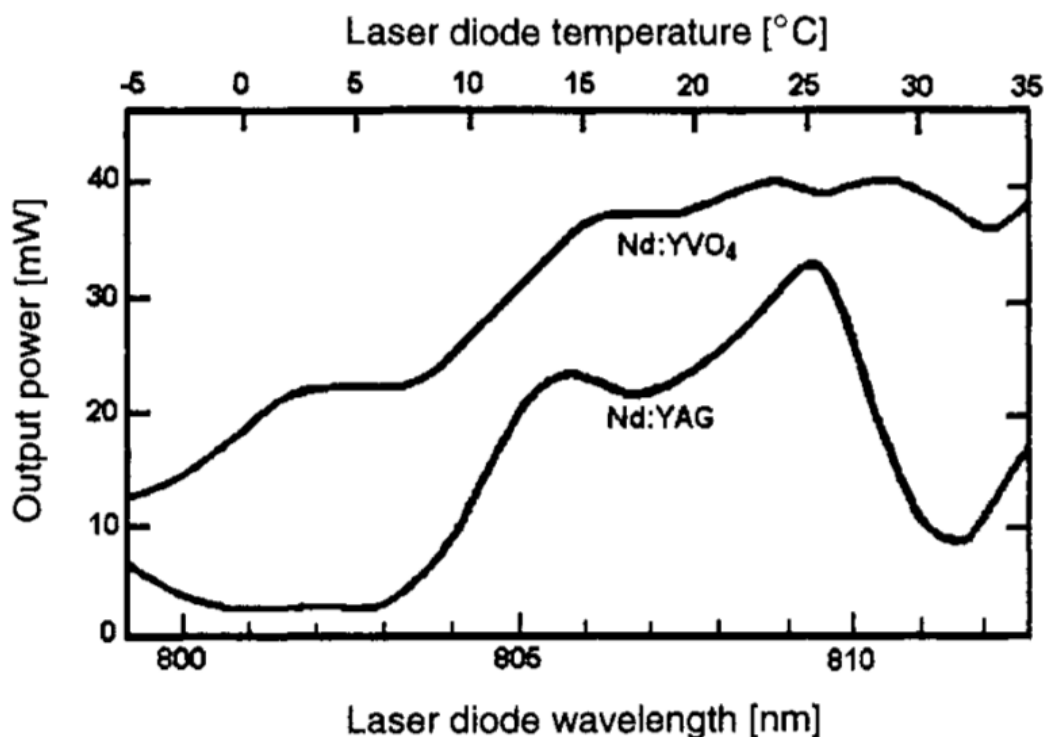
Obrázek 3.2: Výstupní výkon \text{Nd:YVO}_4 laseru v závislosti na teplotě diody a vlnové délce [2].
