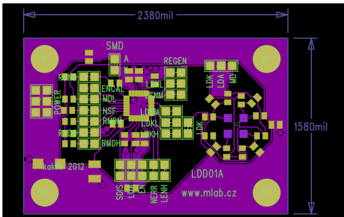
Obrázek 3.12: Návrh plošného spoje pulzního budiče čerpačí diody
