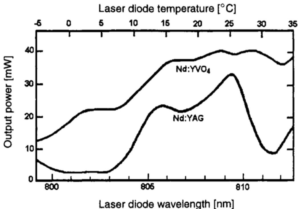
Obrázek 3.2: Výstupní výkon typického \text{Nd:YVO}_4 laseru v závislosti na teplotě diody a vlnové délce [2].
