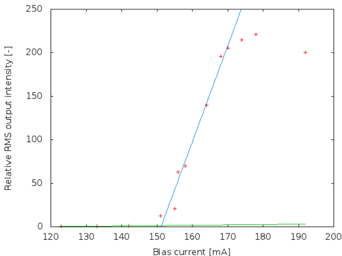
Obrázek 9: Závislost intenzity výstupního záření na proudu čerpací diodou.
