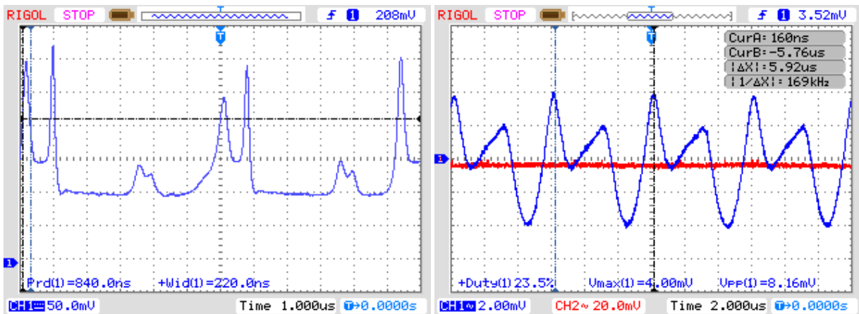
Obrázek 11: Průběh výstupních impulzů v případě použití 5mW verze modulu.
