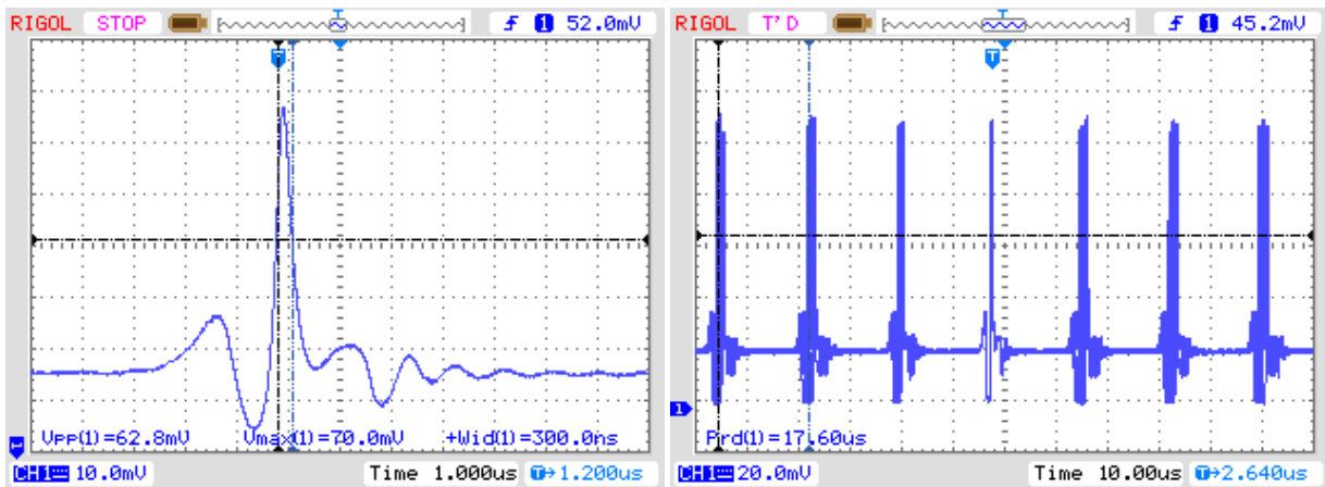
Obrázek 10: Časové průběhy výstupních impulzů laseru pro 20mW modul s vhodně nastaveným pracovním bodem.
