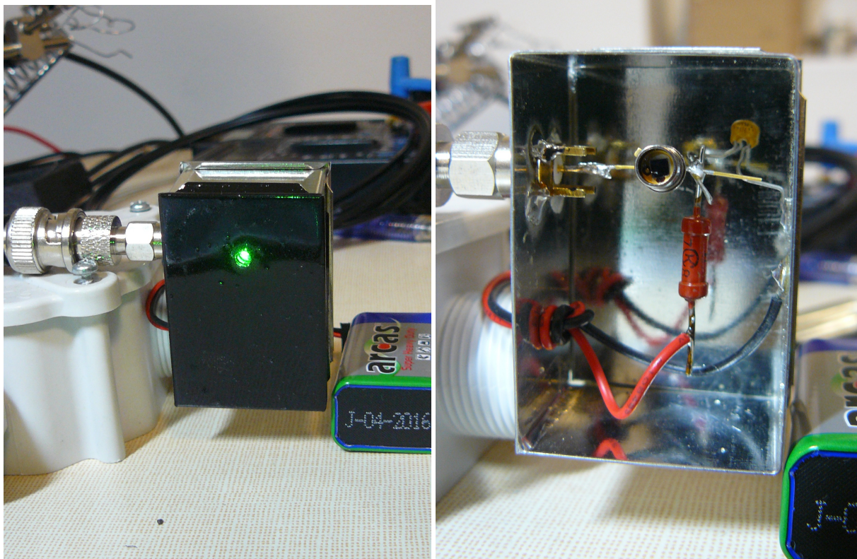
Obrázek 8: Realizovaný detektor časového průběhu záření
