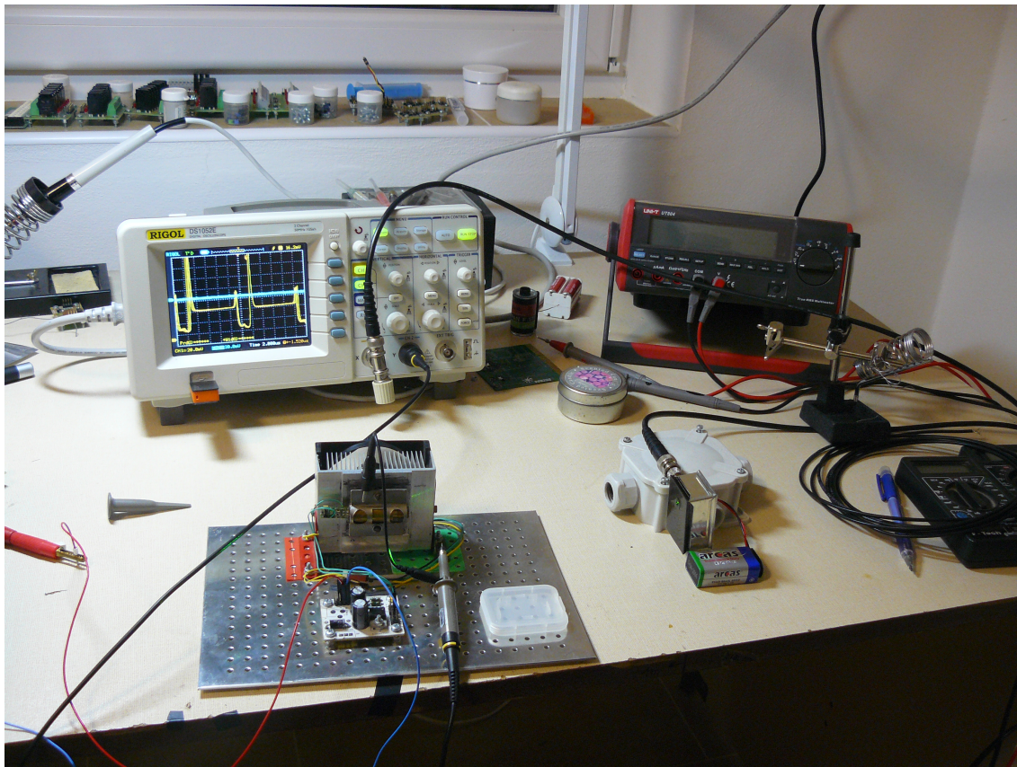
Obrázek 5: Měření prováděné s původním regulačním obvodem.
