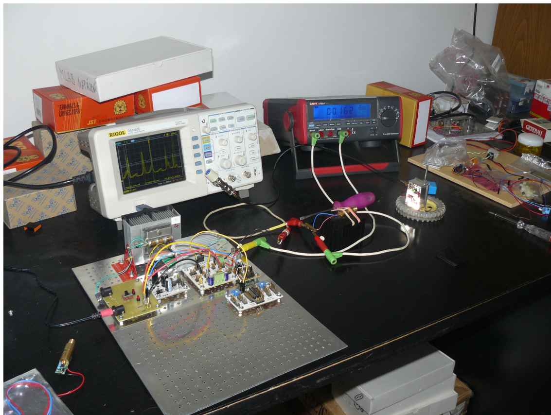
Obrázek 12: Aparatura použitá pro měření intenzity optického výstupu v závislosti na budícím proudu.
