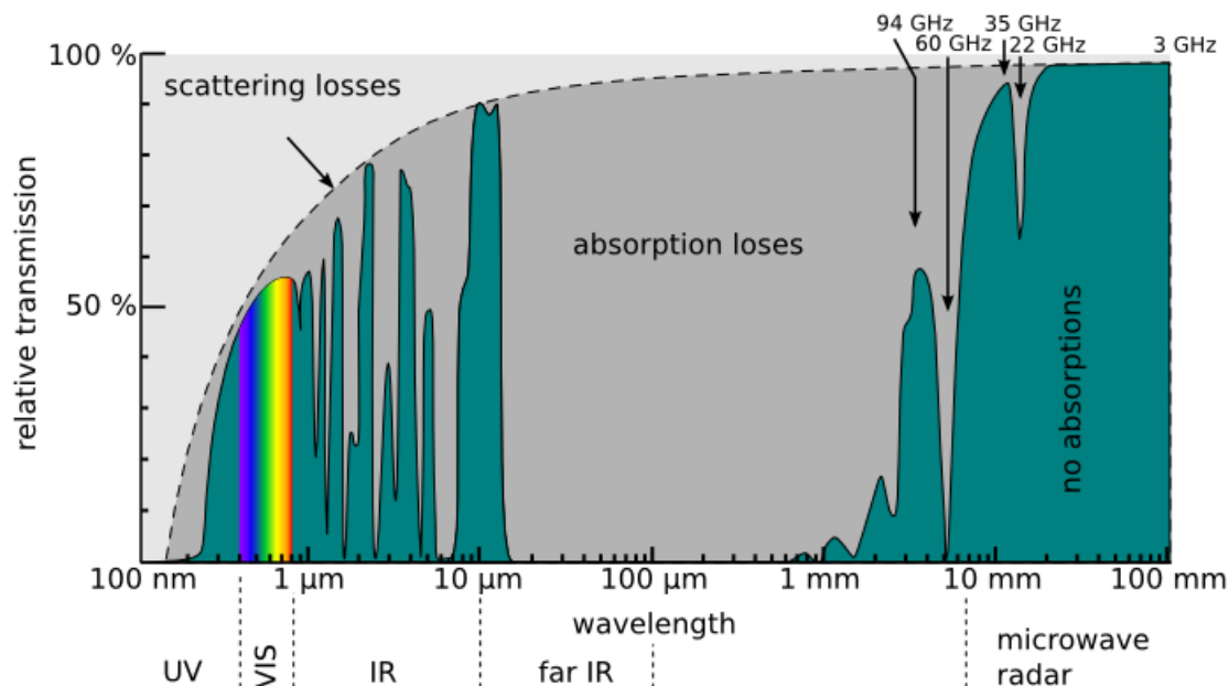
Obrázek 1: Závislost transmisivity čisté atmosféry na vlnové délce záření
