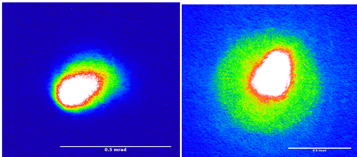
Obrázek 4: Promítané stopy svazků ve vzdálenosti 20m od modulu. Vlevo modul 5mW, napravo varianta 20mW. Měřítka vpravo dole má rozměr 0,5mrad.
