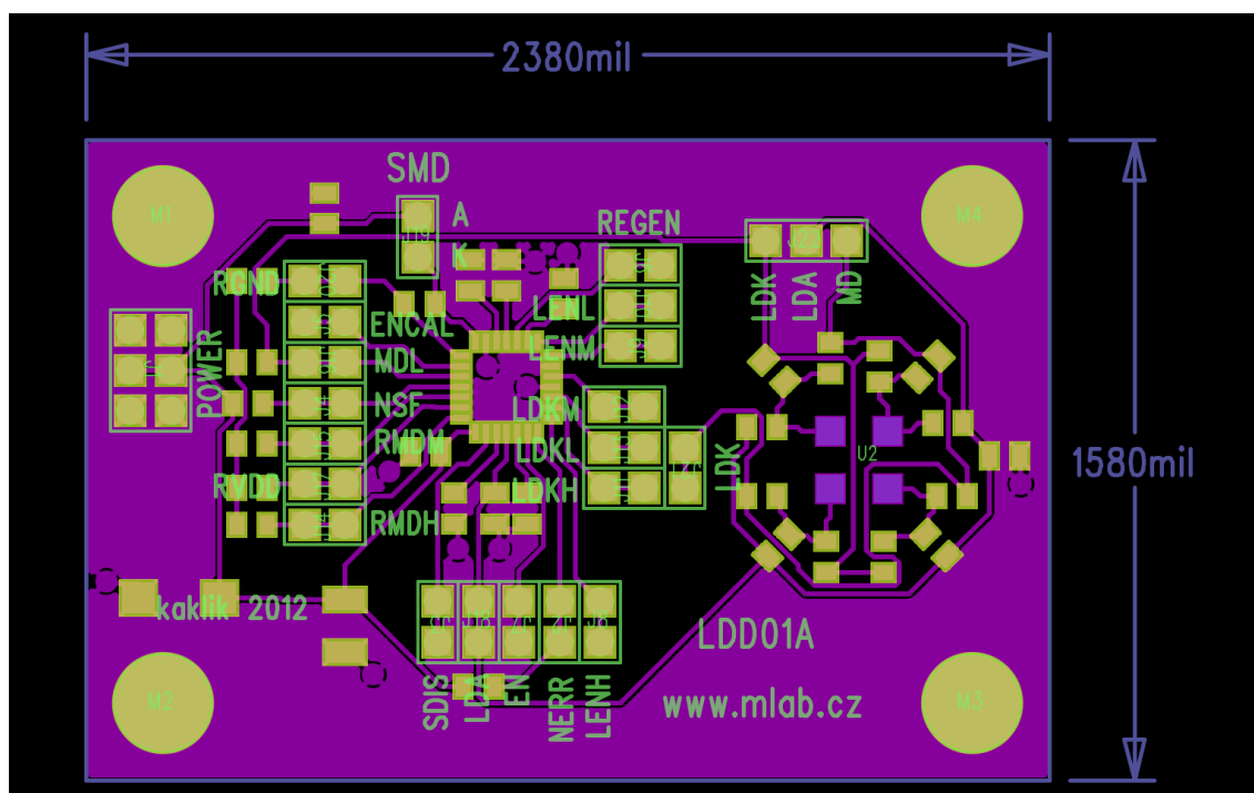
Obrázek 3.12: Návrh plošného spoje pulzního budiče čerpací diody
