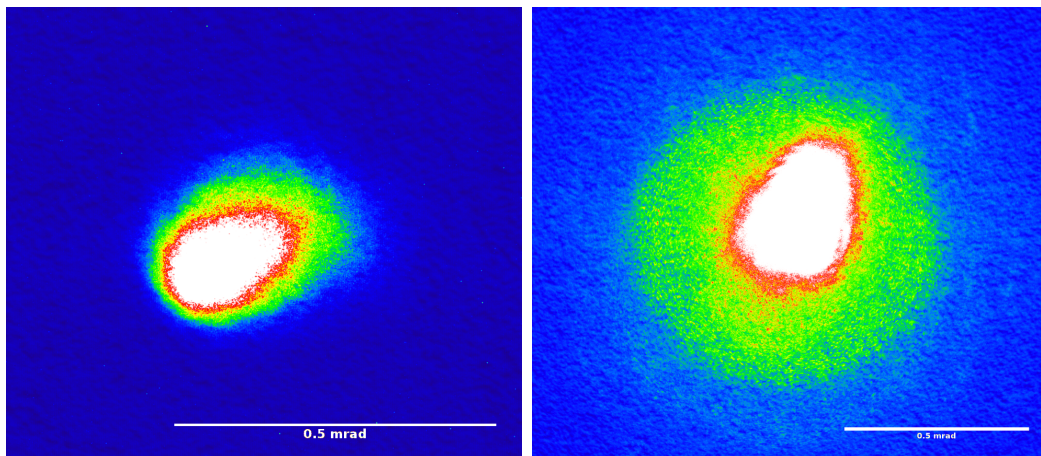
Obrázek 3.3: Promítané stopy svazků ve vzdálenosti 20m od modulu. Vlevo modul 5mW, napravo varianta 20mW. Měřítko vpravo dole má rozměr 0,5mrad.
