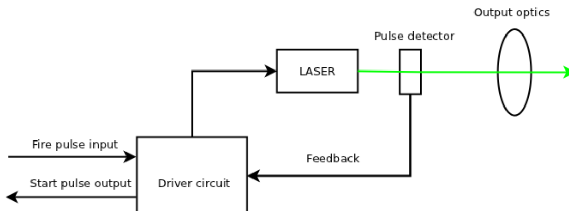
Obrázek 2: Zjednodušené blokové schéma laserového vysílače.
