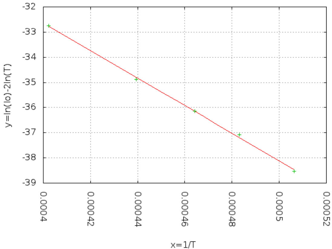
Obrázek 2: Naměřené hodnoty emisního proudu v nasycené oblasti
