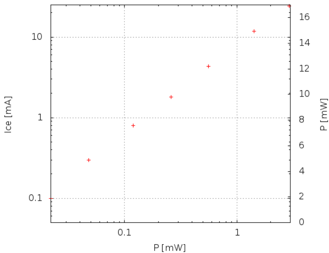
Obrázek 6: Proud protékající fototranzistorem v závislosti na výkonu dopadajícího záření
